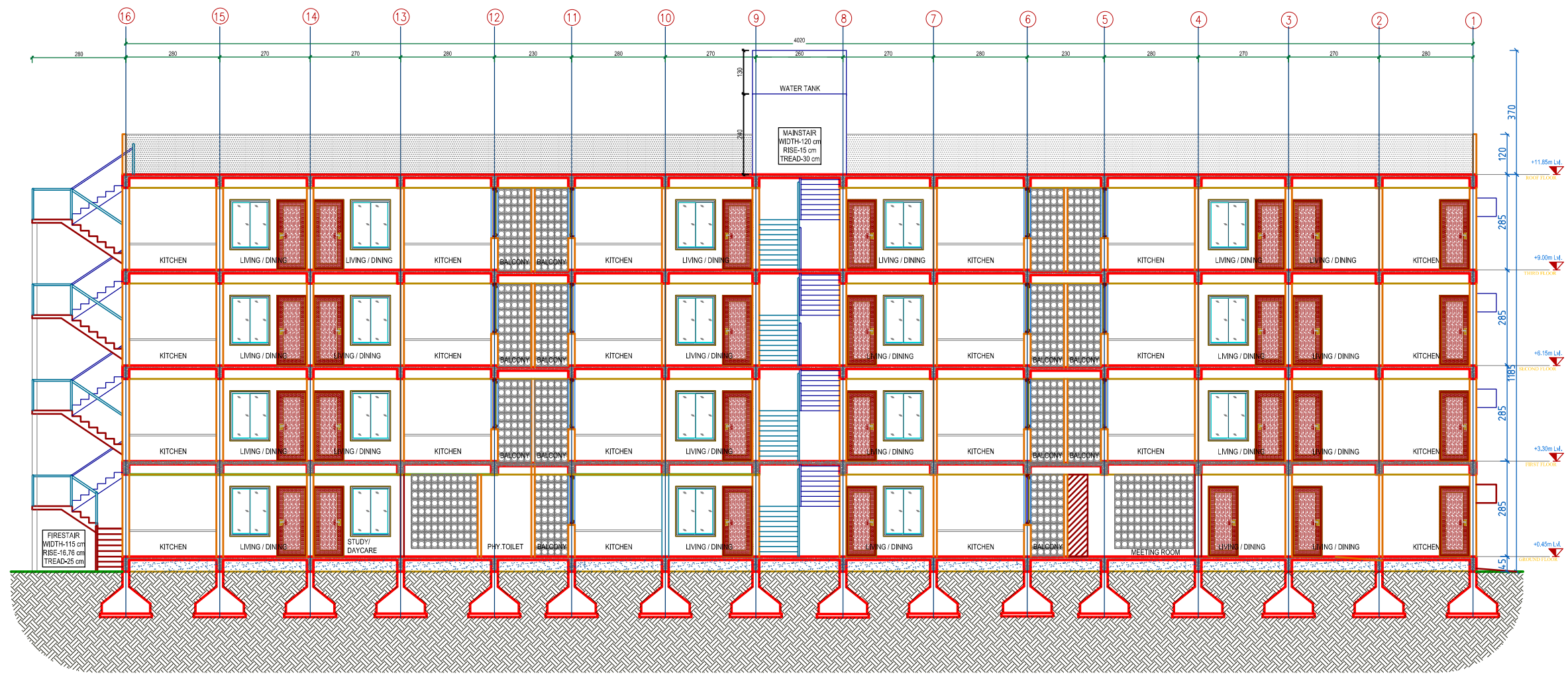
SECTION A-A
